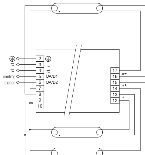
PCA T8 EXCEL one4all lp xitec 3x18W
