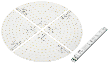
TW CLE 261mm 4600lm 927-965 SELV PRE2
