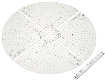
TW CLE 401mm 9800lm 927-965 SELV PRE2
