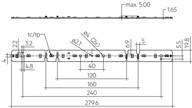
LLE 20x280mm 750lm LV MD ADV1
