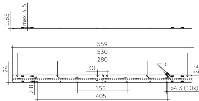
LLE 24x560mm 2200lm 927-965 LV PRE3
