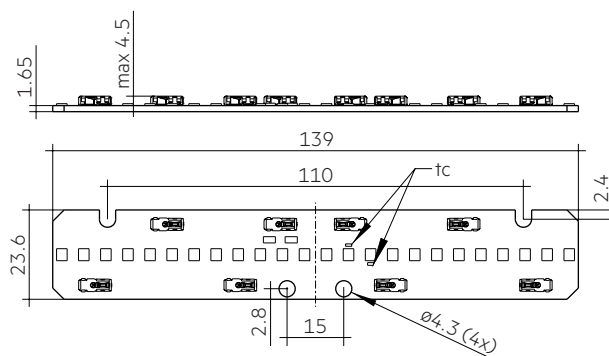
LLE 24x140mm 550lm 927-965 LV PRE3
