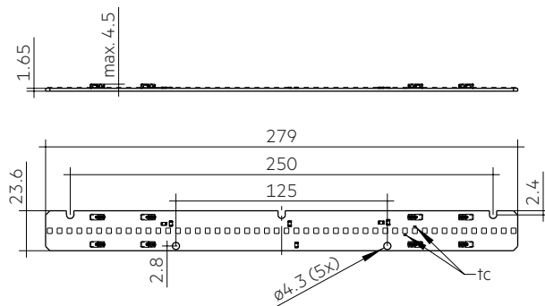
LLE 24x280mm 1100lm 927-965 LV PRE3
