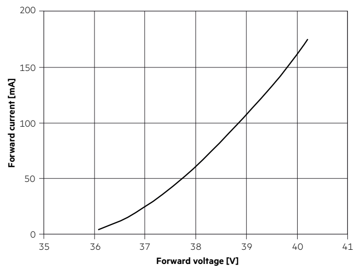
LLE 24x280mm 750lm 9xx LVD ADV1
