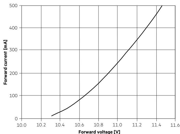
LLE 24x280mm 650lm 9xx HV ADV5
