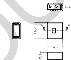
ACL plug end cap IP67
