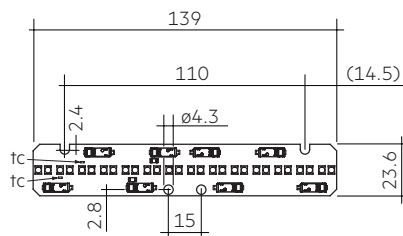
LLE G2 24x140MM 750LM 927-965 LV PRE
