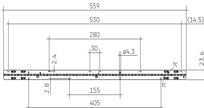
LLE G2 24x560MM 3000LM 927-965 LV PRE
