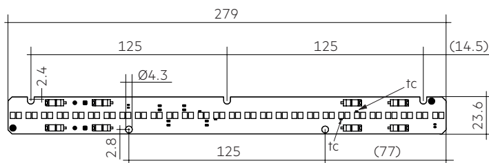
LLE G2 24x280MM 1500LM 927-965 LV PRE
