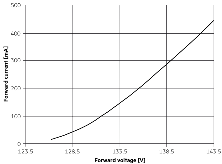
LLE G4 24x1120mm 8000lm 8x0 ADV
