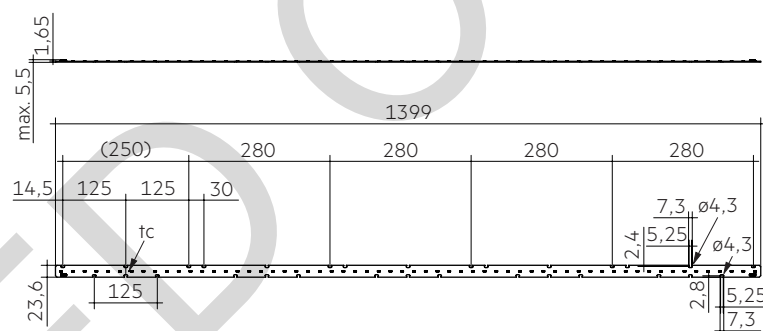
LLE G4 24x1400mm ADV
