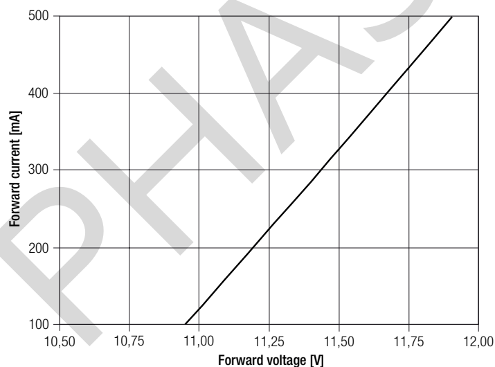
LLE G4 24x280mm 650lm 8xx ADV
