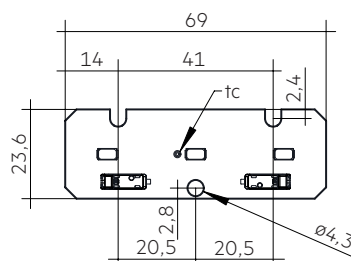
LLE G4 24x70mm 160lm ADV
