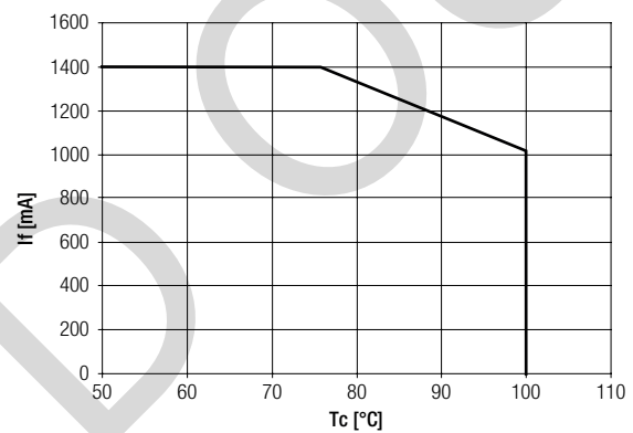
SLE G5 23mm 6000lm 927 EXCITE
