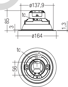
DLA G1 150mm 2000lm 8xx R SH SNC
