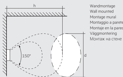
smartSWITCH HF 5DP S f (28002235)
