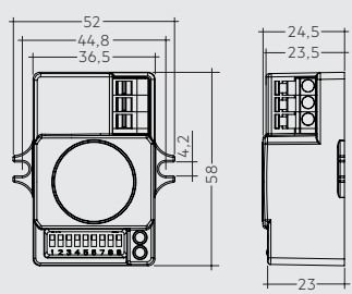
smartSWITCH HF 5DP S f (28002235)
